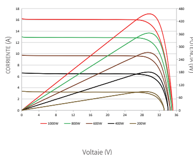
Curvas de corriente-voltaje y potencia-voltaje (445W)
